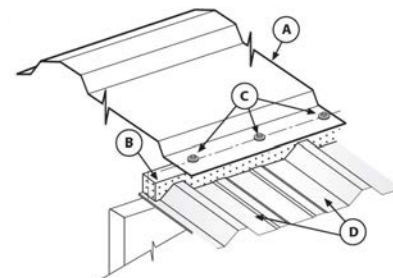
EXEMPLE DE MONTAGE QUI S'APPLIQUE AUX 2 PROFILS AVEC FAITIÈRE STANDARD
